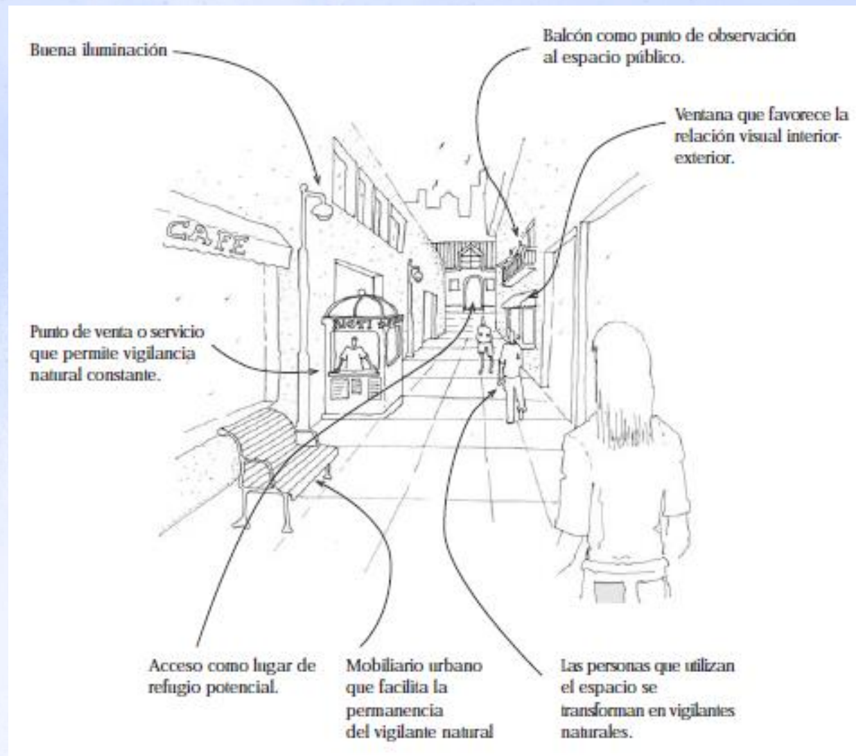
Fig. 10 b Si la estructura de la vivienda y normativas lo permiten, se recomienda ampliar ventanas.
